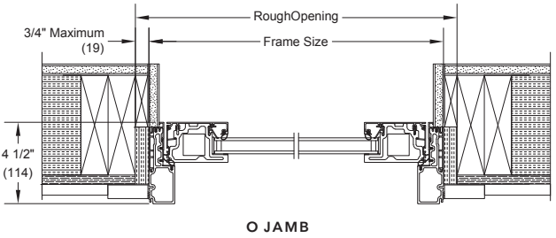
O JAMB
