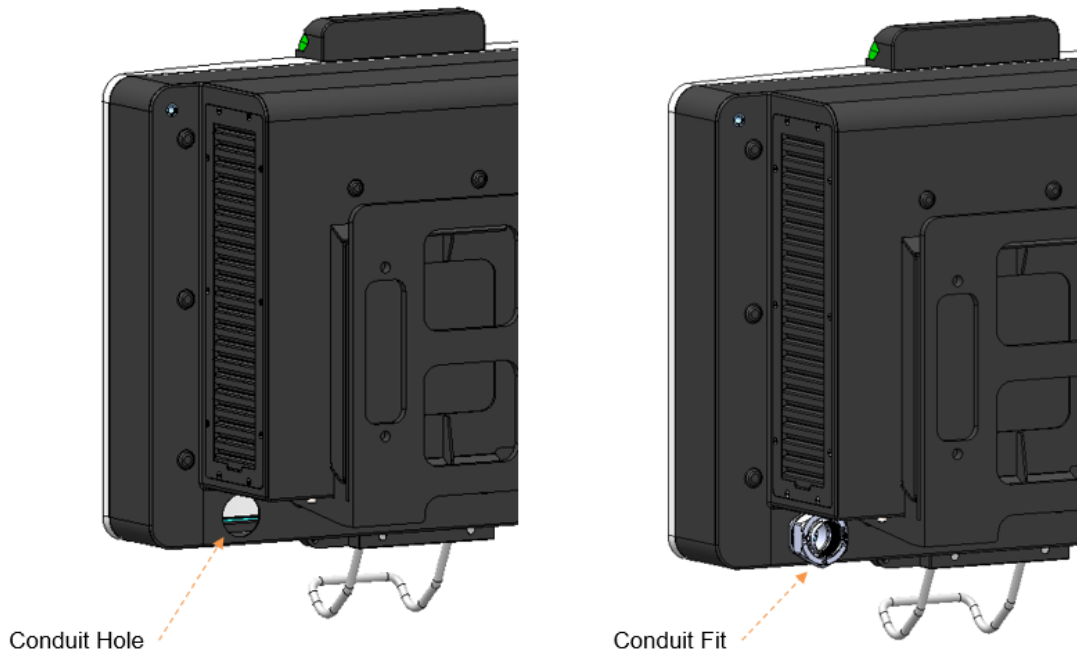
Fig. 43 – Attach conduit fitting
