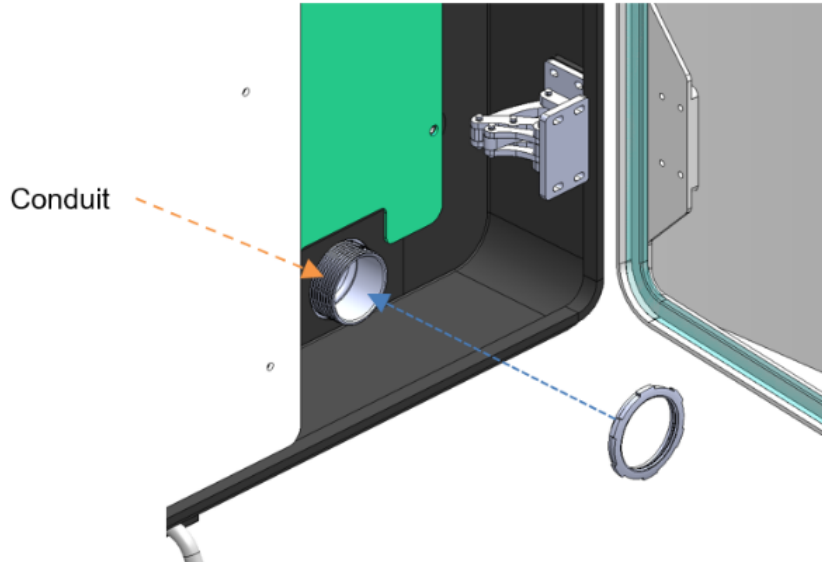
Fig. 30 – Attach conduit fitting
